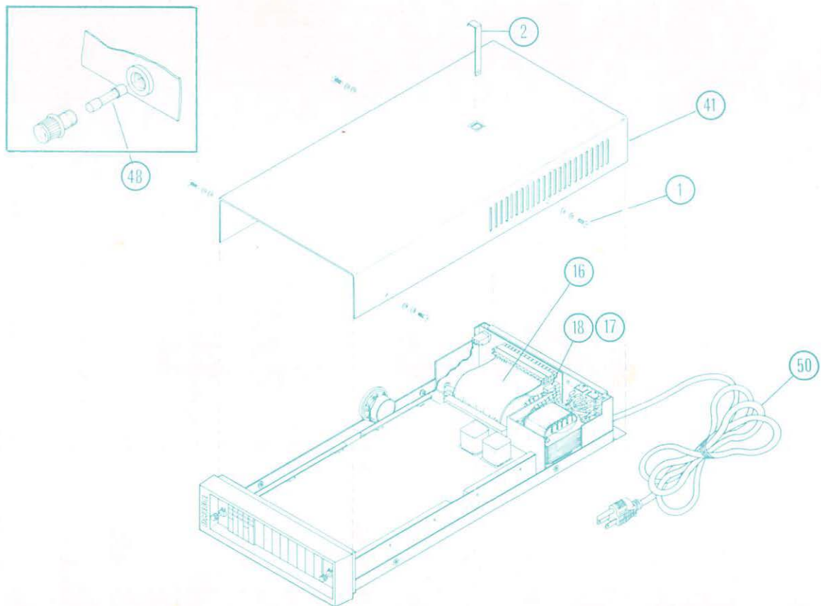
Fig. : 1.1 : Caixa RT - Vista explodida 1
