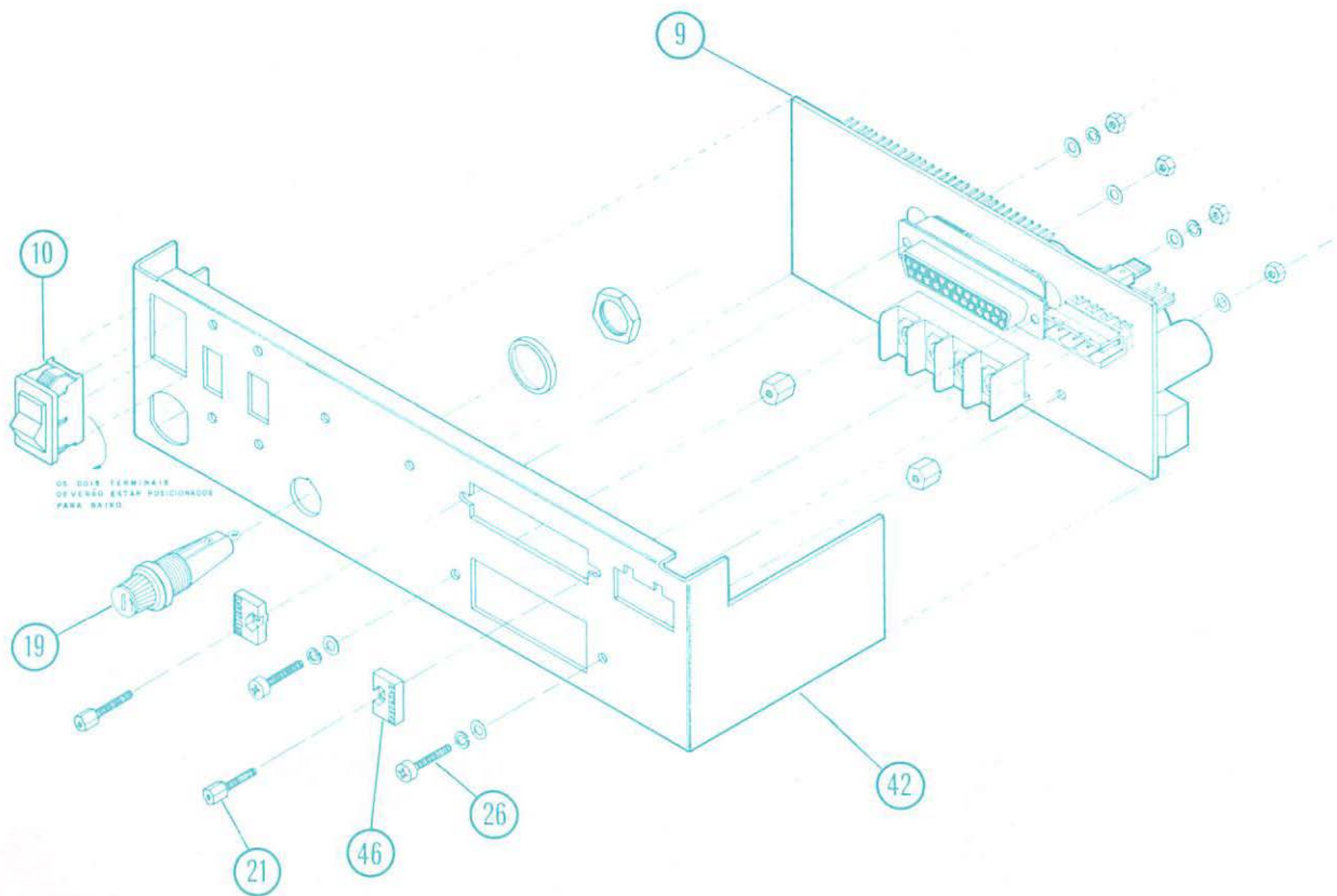
Fig. : 1.4 : Caixa RT - Vista explodida IV
