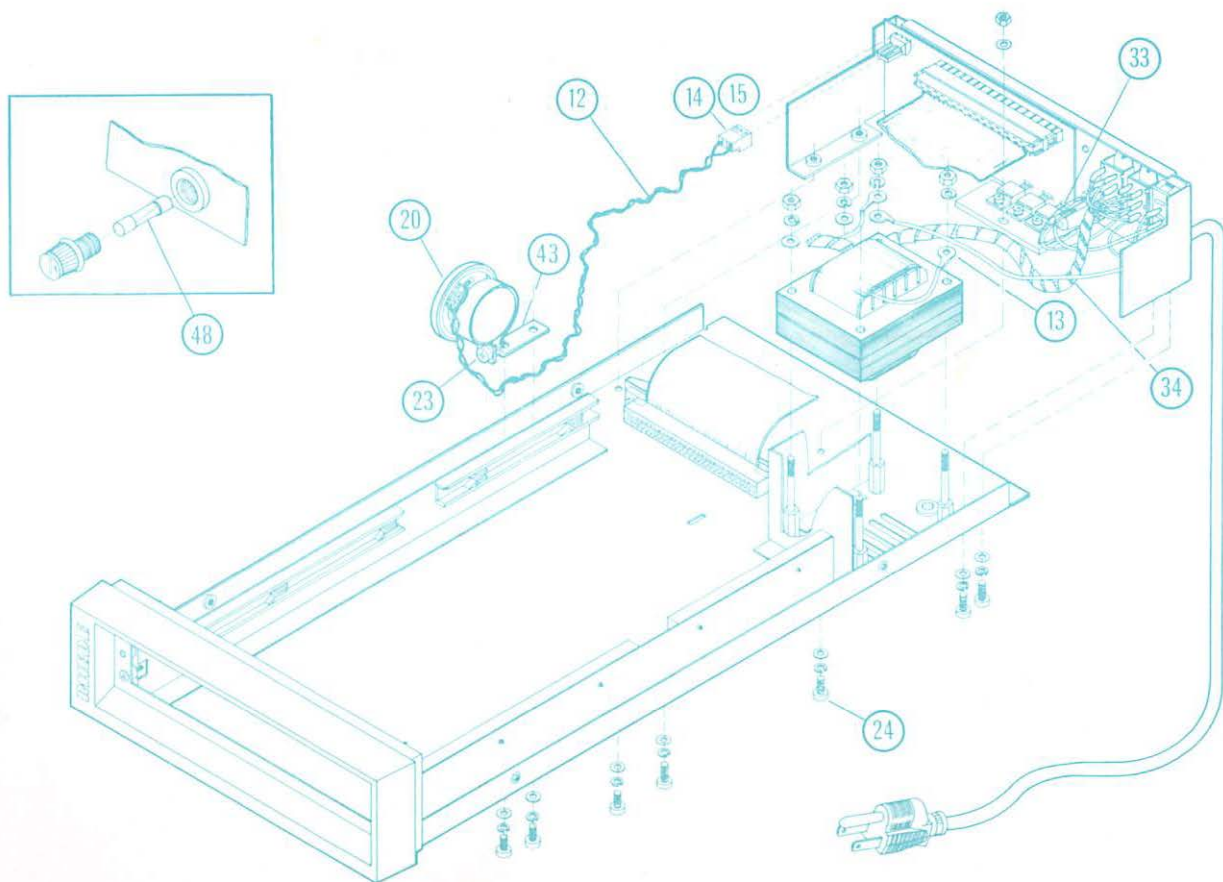
Fig. 1.2 : Caixa RT - Vista explodida II
